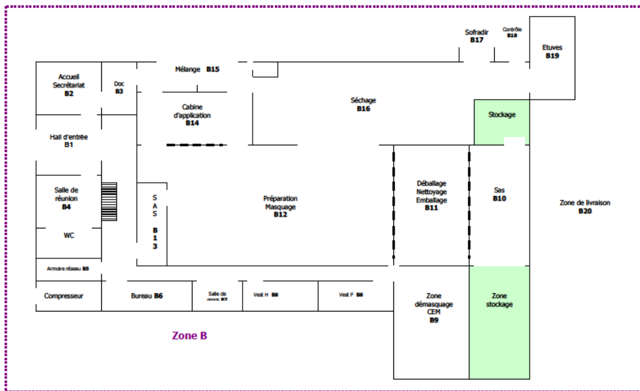
Plan du site 2 Juillet 2000 - Révision 1a - vérifier la validité de la révision de ce document avant toute utilisation Page 1 sur 1 MAP Plan du site Pamiers 2 Définition des unités de travail
